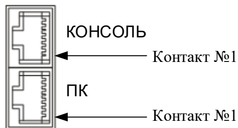
Цоколевка разъемов «ПК» и «Консоль» (вид со стороны задней стенки)
