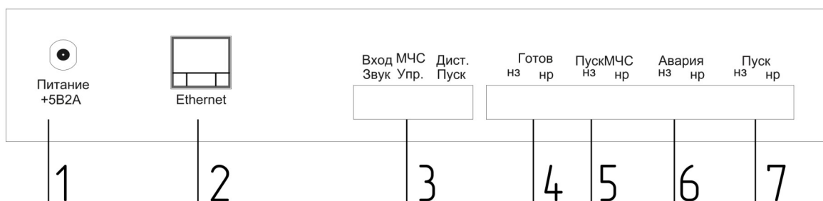
Рисунок 2 - Вид сзади
