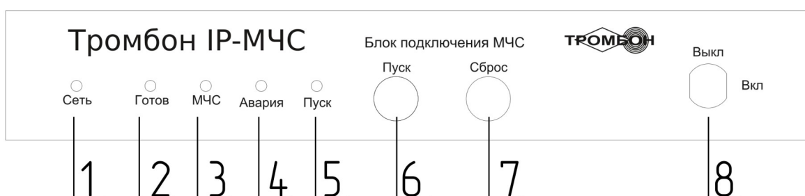
Рисунок 1 - Вид спереди
