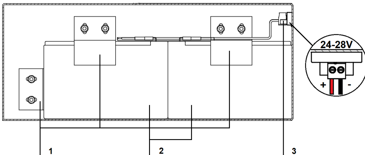
Рисунок 3 - Отсек установки аккумуляторных батарей. Размещение АКБ
