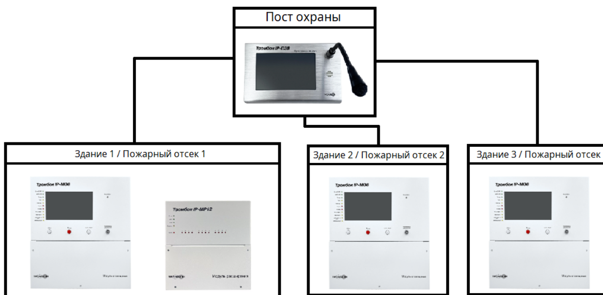
Рисунок 16 - Деление системы на пожарные отсеки / независимая работа в разных зданиях.
