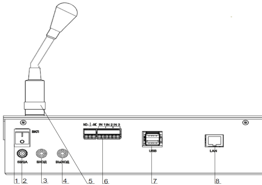
Рисунок 2 - Задняя панель
